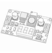
1x 02502 LM2596 Buck Converter
